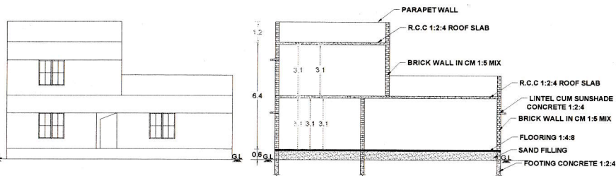
ELEVATION
