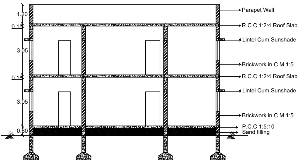
SECTION - AB
