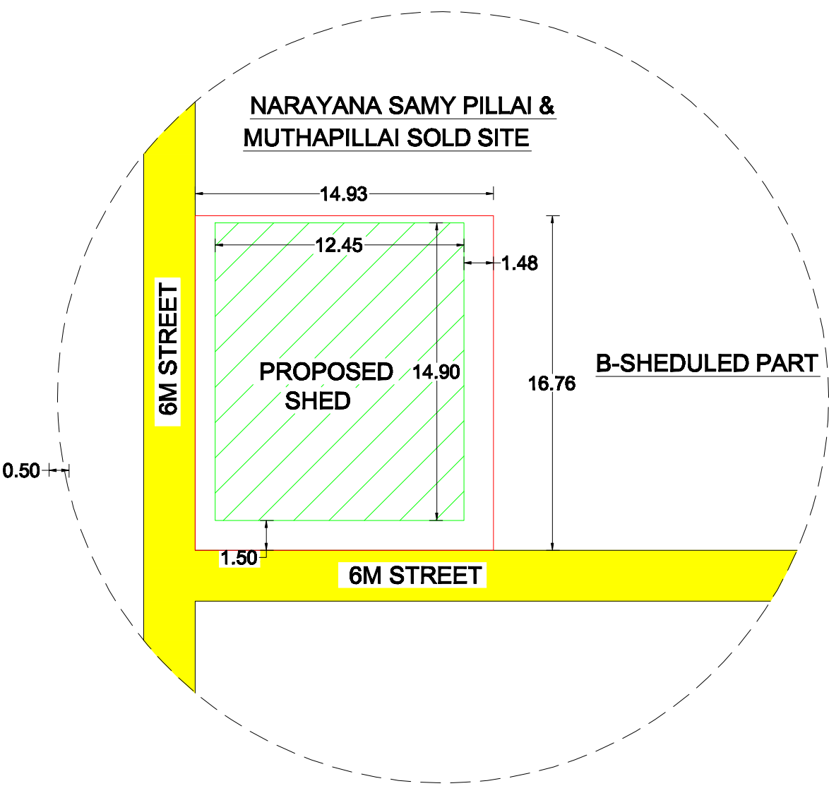
SITE PLAN SALE 1:100
