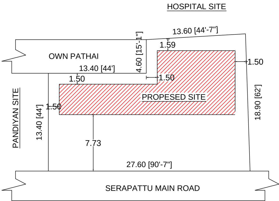
SITE PLAN PLAN SCALE 1:100
