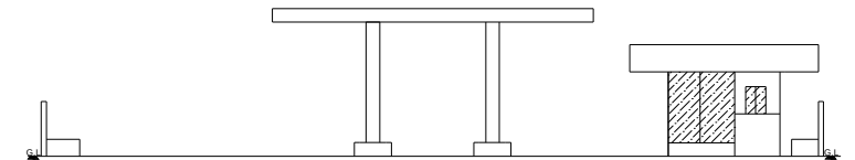
ELEVATION
