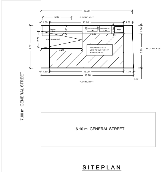
SITEPLAN SCALE 1:100
