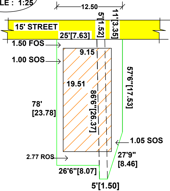
SITE PLAN SCALE : 1:25
