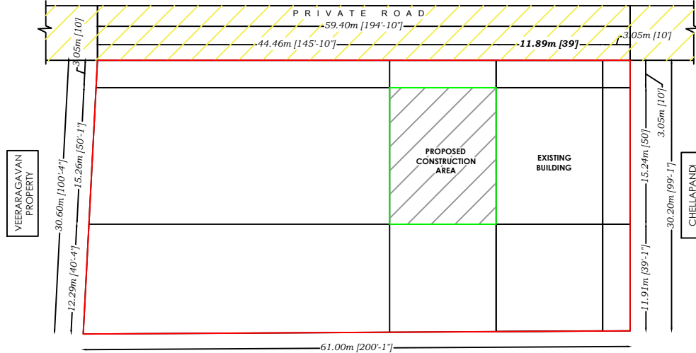
SITE PLAN: 1:100
