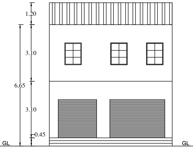
ELEVATION
