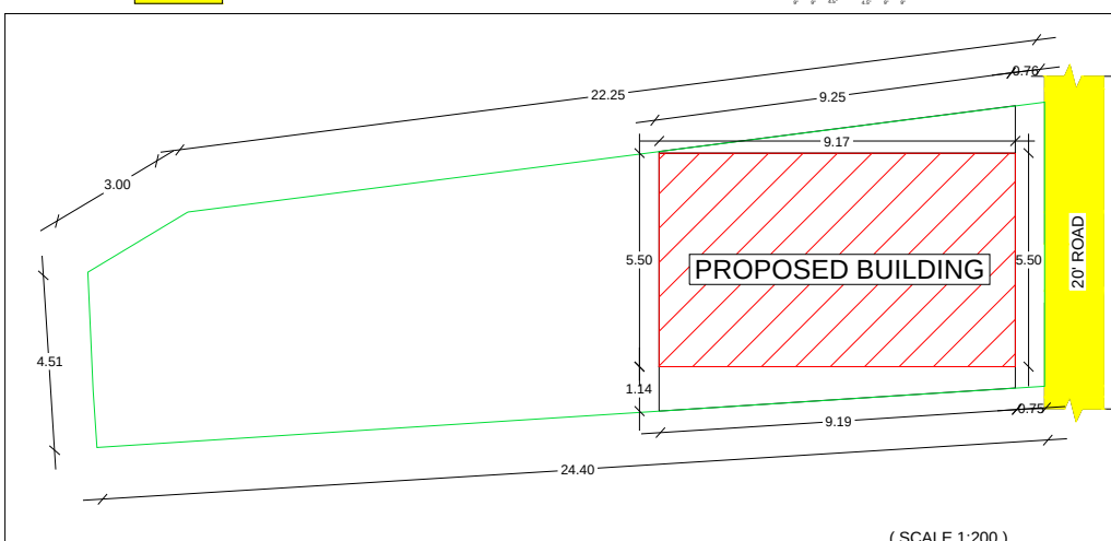
(SCALE 1:200)
