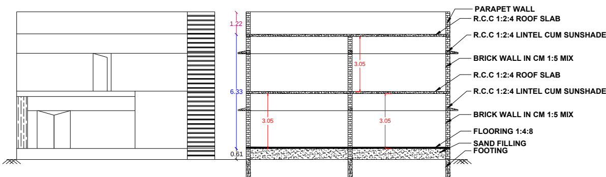
ELEVATION
