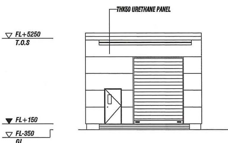
3 ELEVATION SCALE: 1/100
