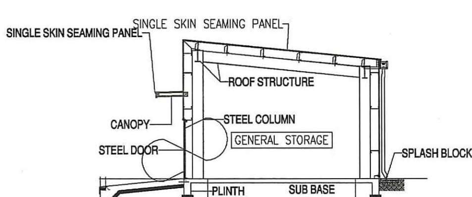
1 SECTION SCALE: 1/100
