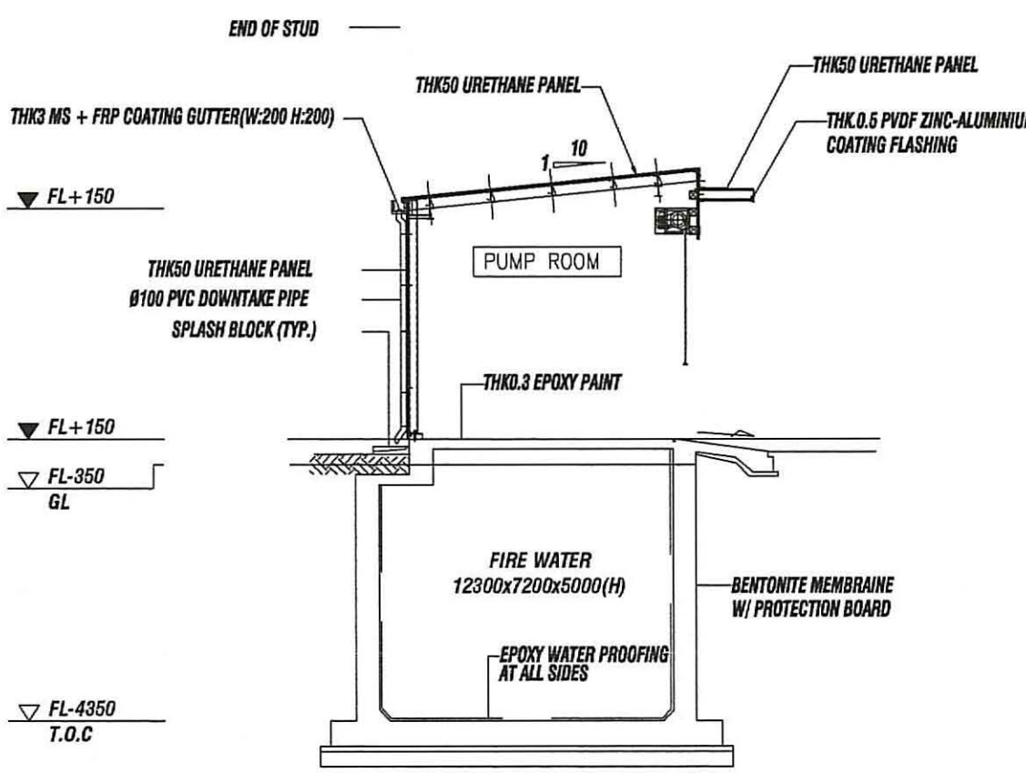
4 SECTION SCALE: 1/100
