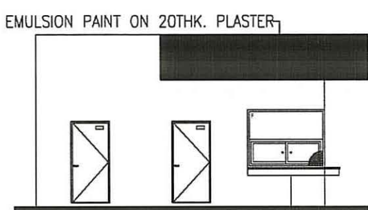
3 ELEVATION SCALE: 1/100
