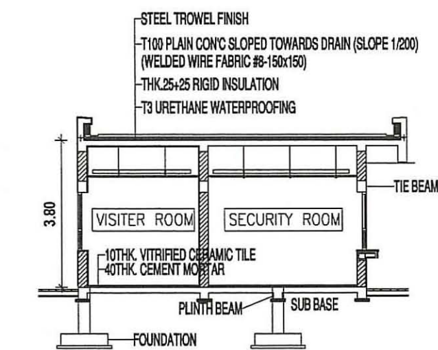
4 SECTION SCALE: 1/100
