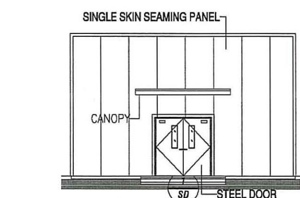
3 ELEVATION SCALE: 1/100
