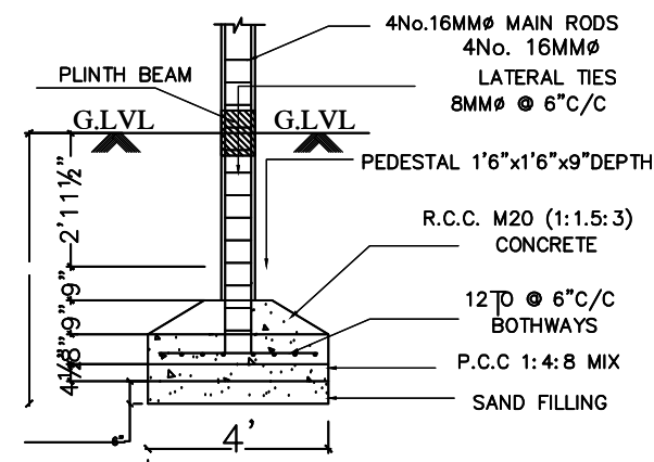
[SCALE: 1:50]
