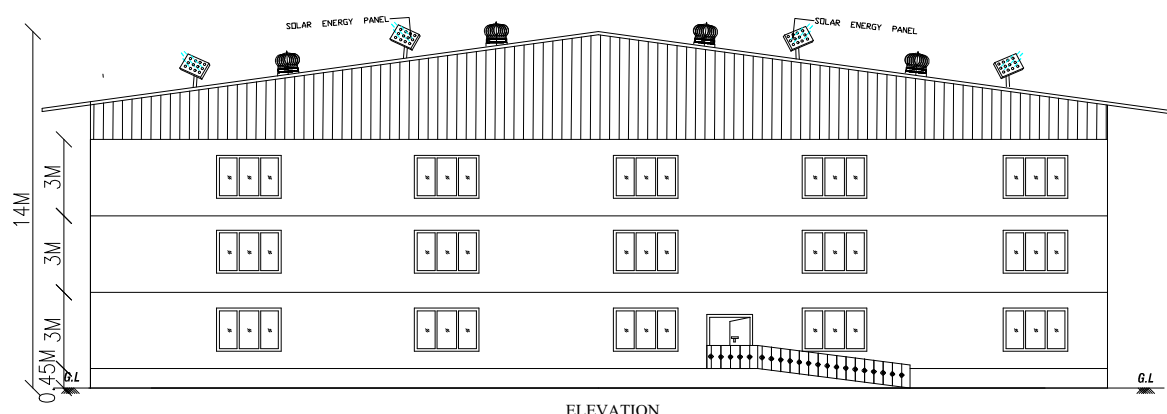
ELEVATION
