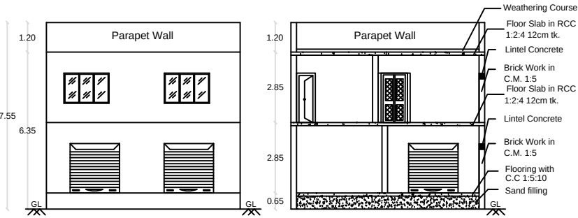
ELEVATION
