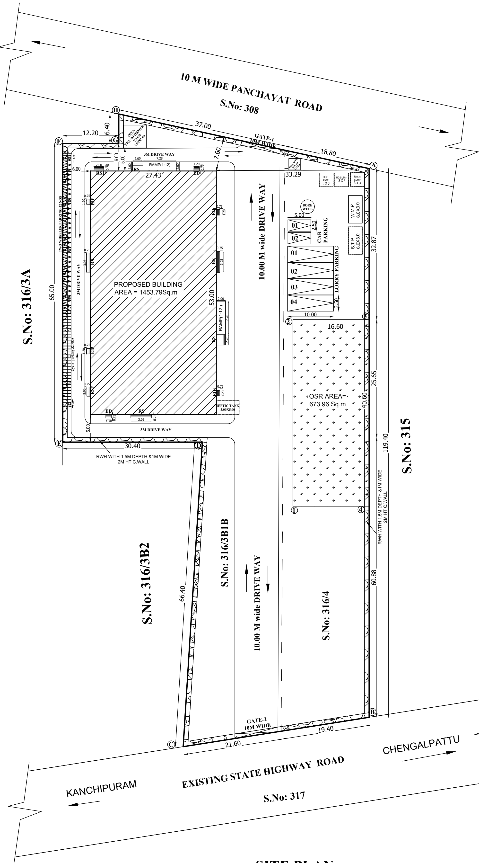
SITE PLAN 1:400
