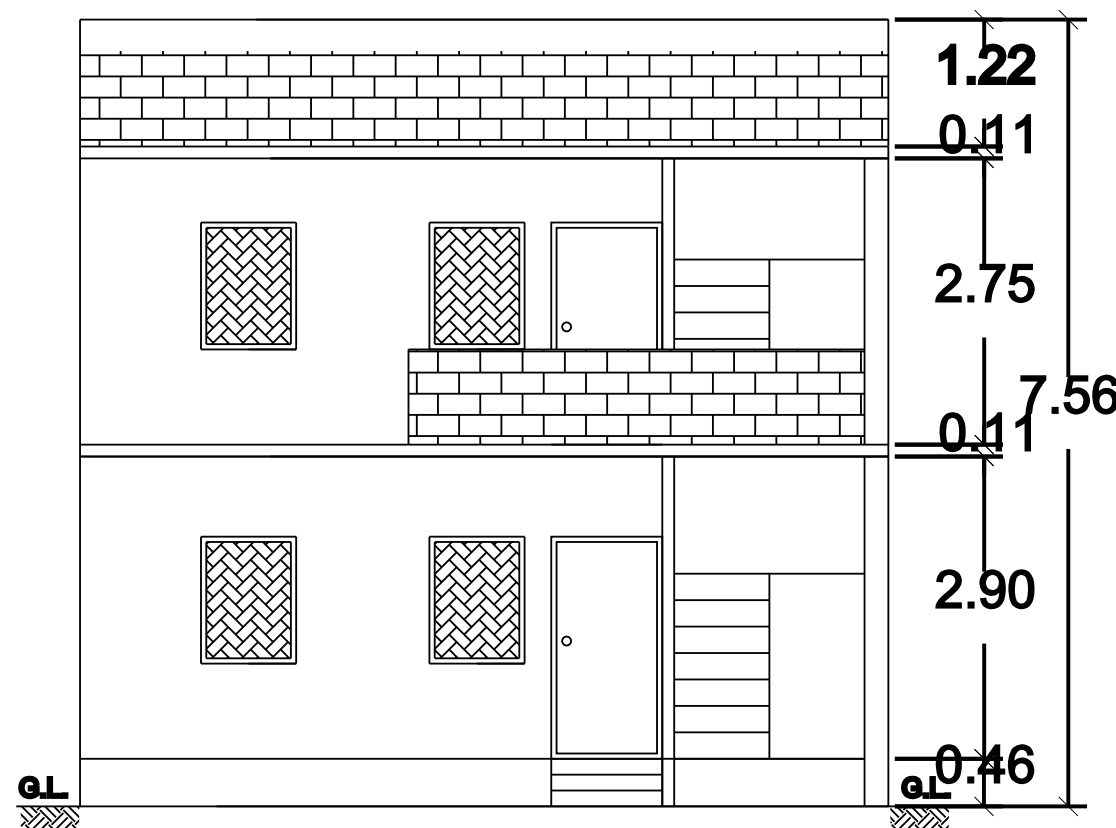
ELEVATION
