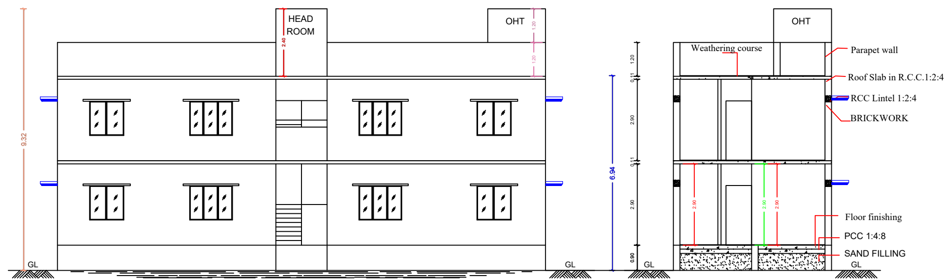
ELEVATION
