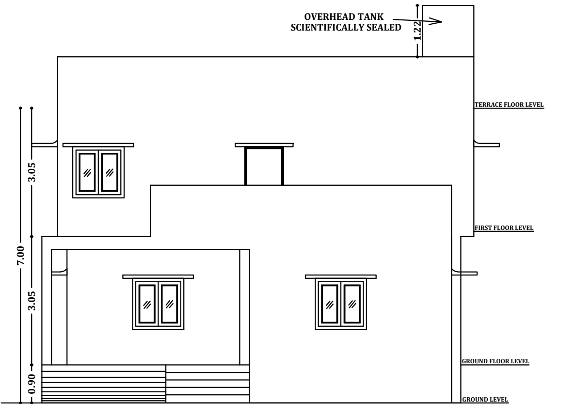
ELEVATION
