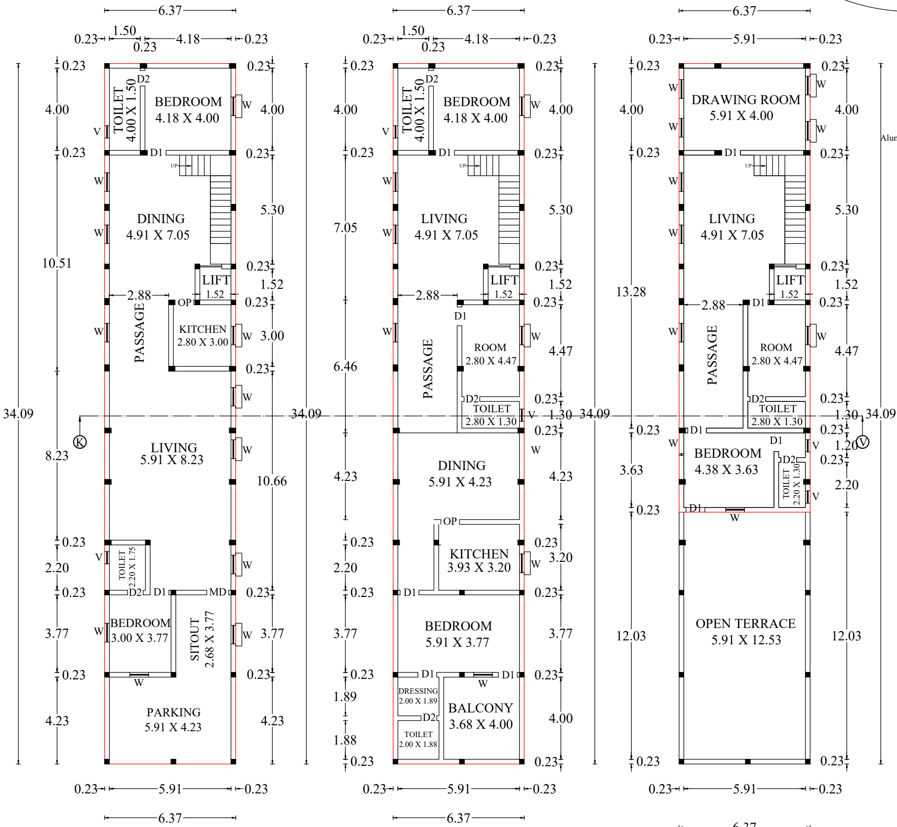
PRO. G. F. PLAN
