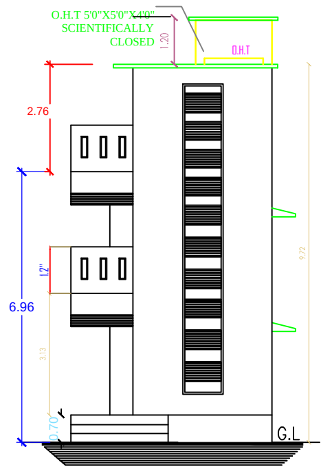
ELEVATION
