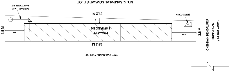
SITE PLAN ( SCALE 1:100 )
