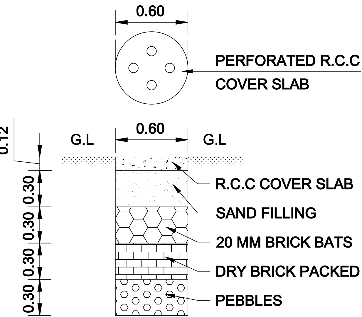
ELEVATION
