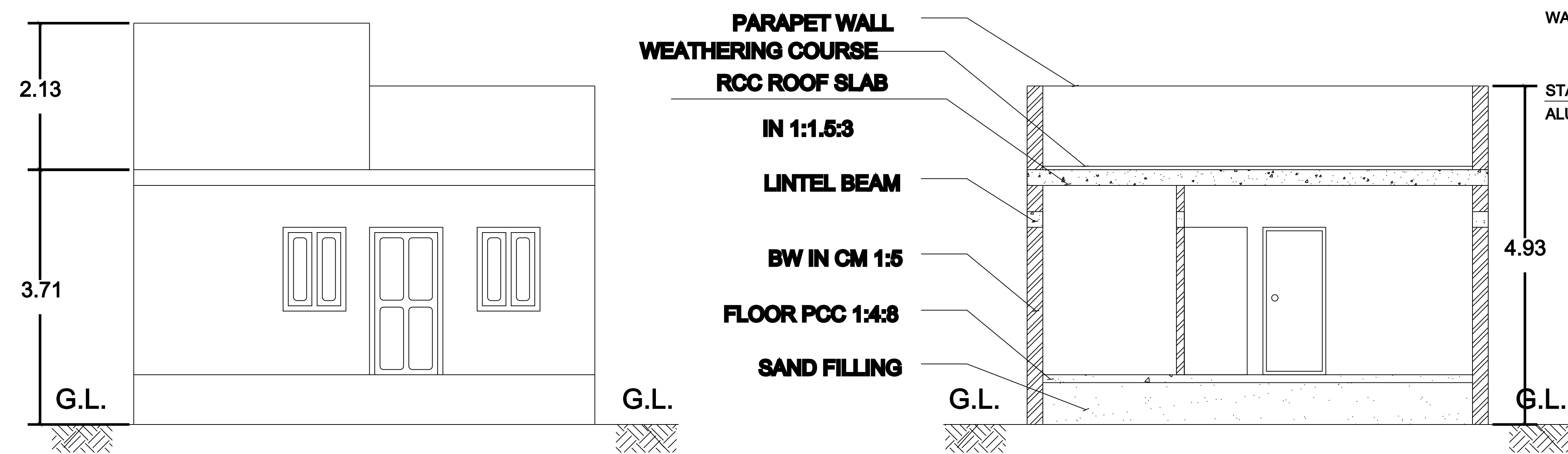
ELEVATION
