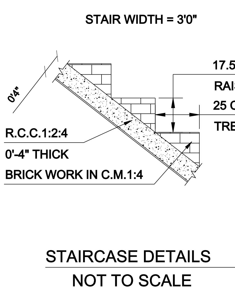
SECTION E-V
