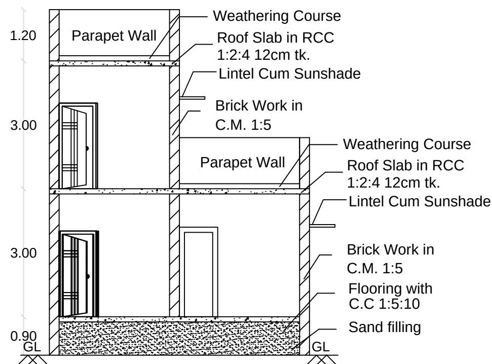
SECTION A-B
