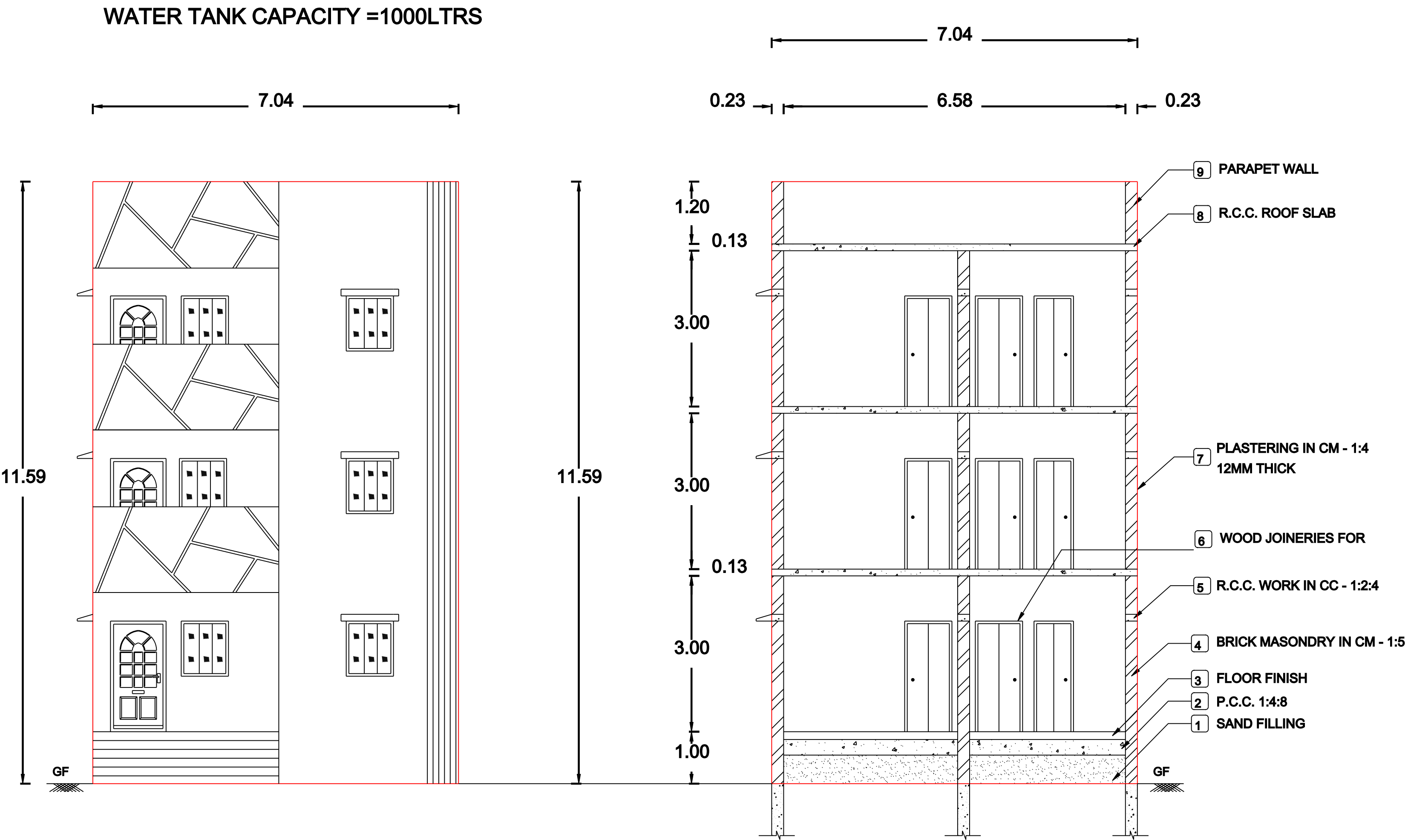
ELEVATION
