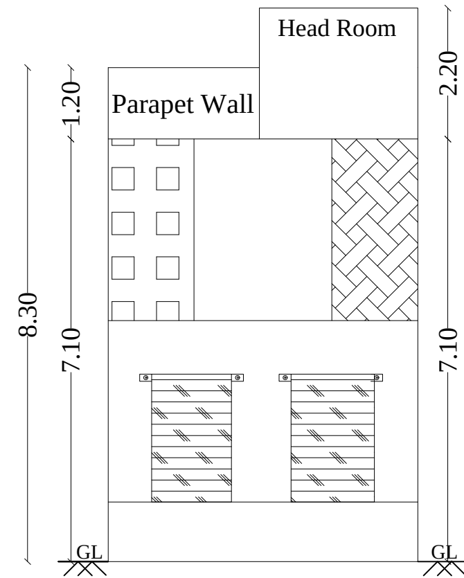
ELEVATION
