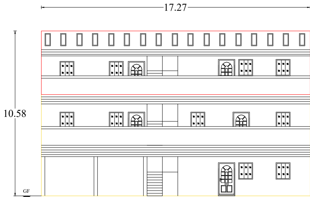
ELEVATION
