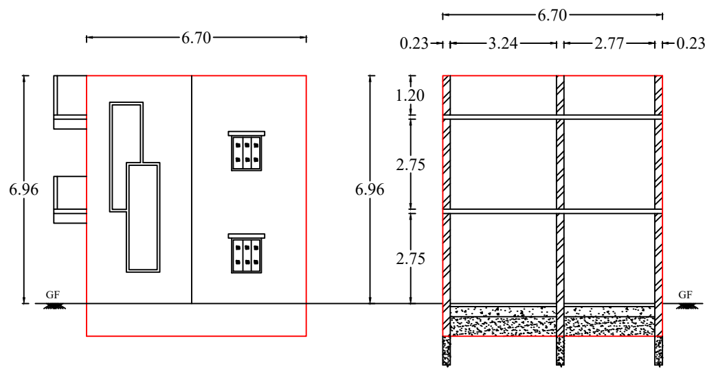
ELEVATION
