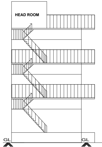
ELEVATION
