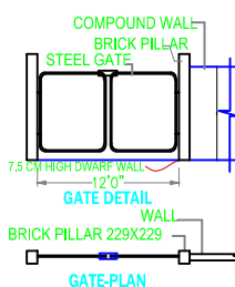
GATE-PLAN
