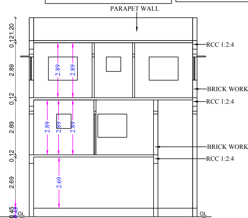
SECTION - AB
