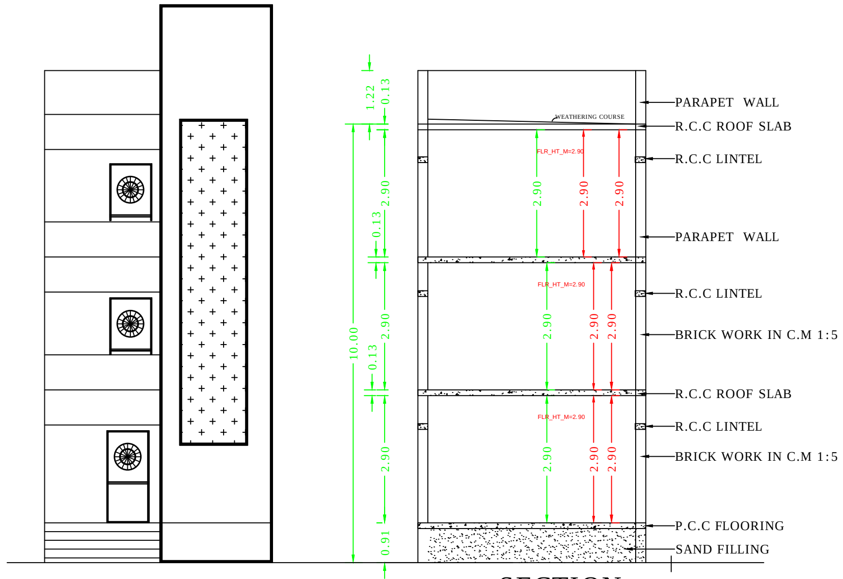
ELEVATION
