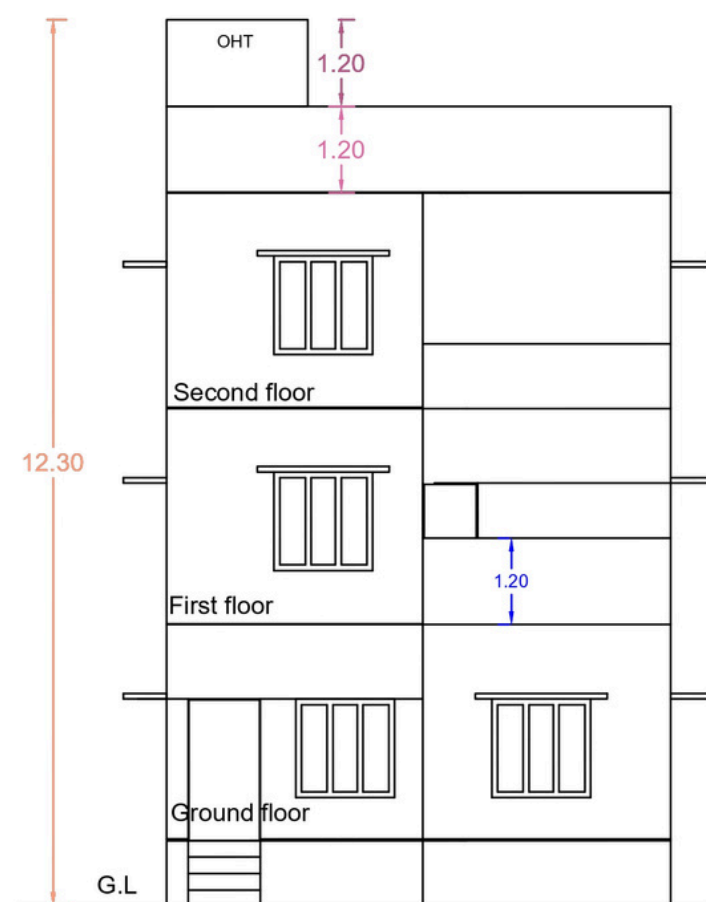
ELEVATION
