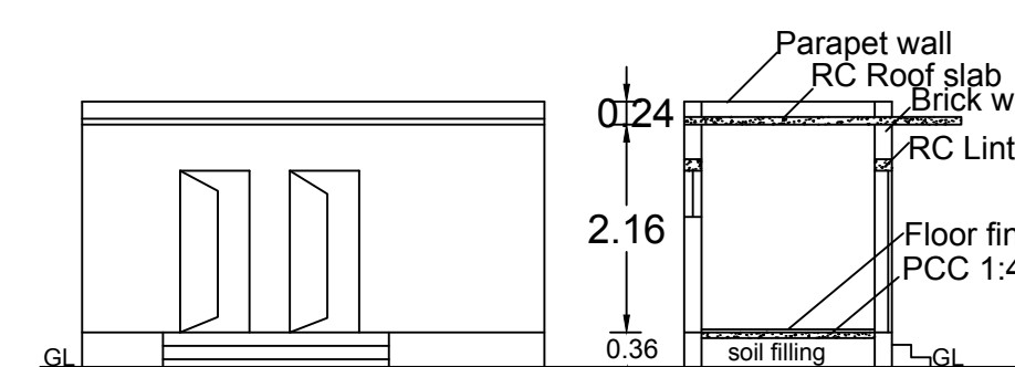
ELEVATION
