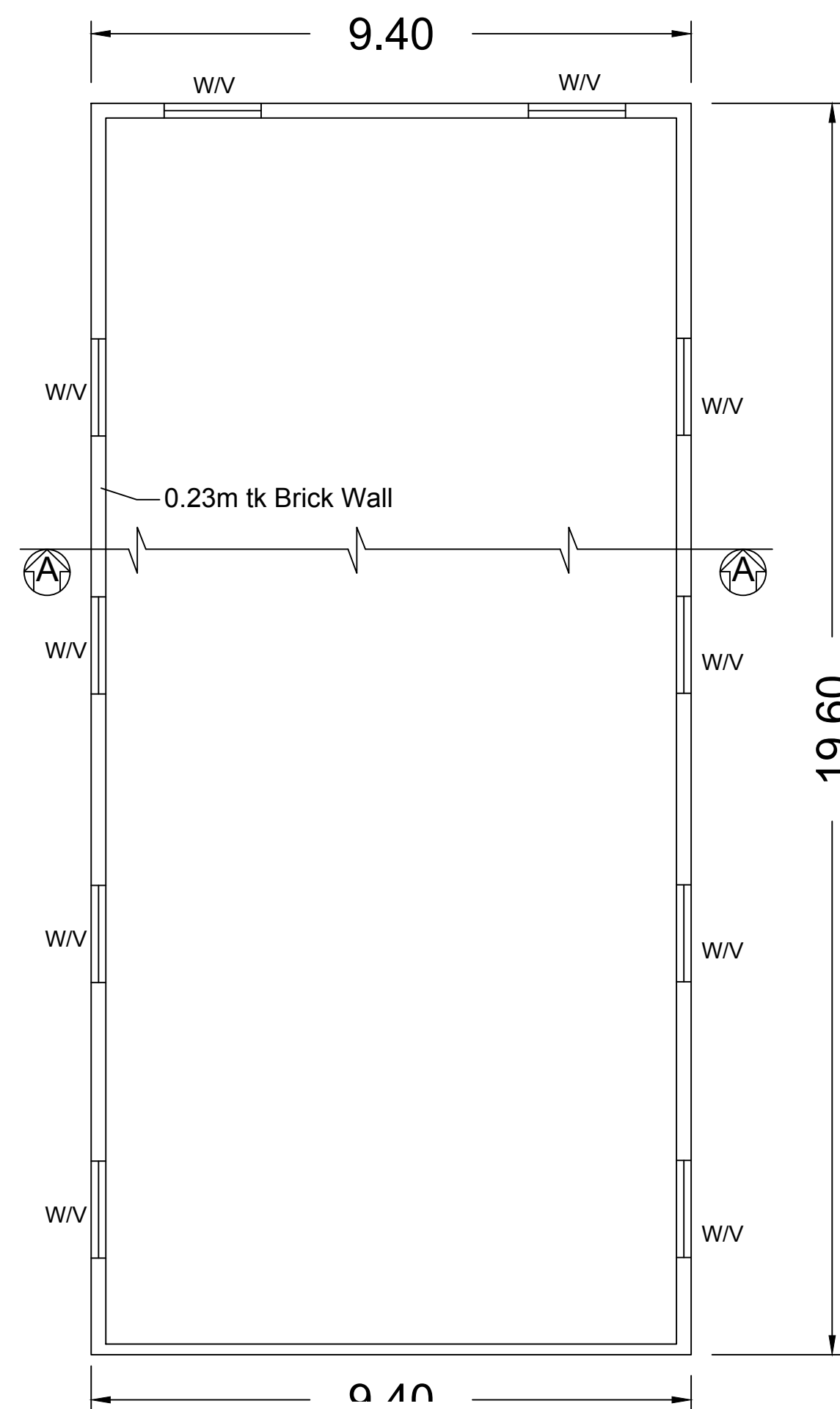
D PLAN
