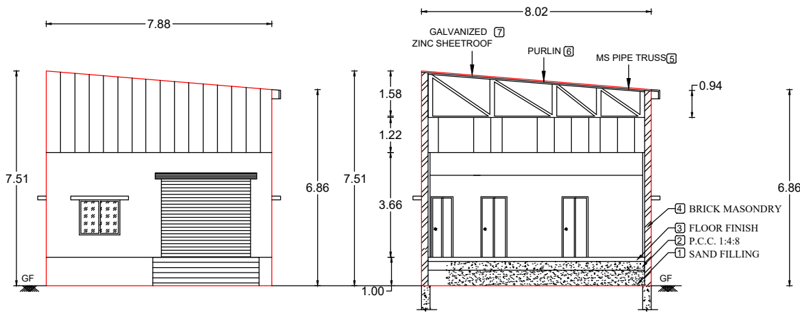
ELEVATION
