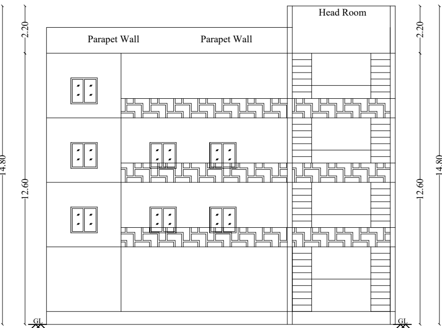
ELEVATION
