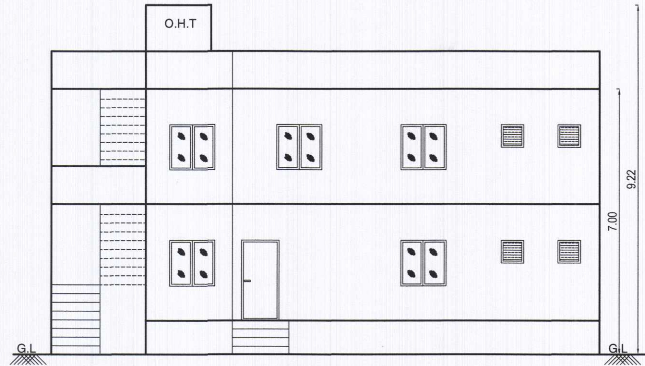
ELEVATION
