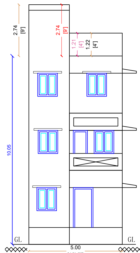
ELEVATION
