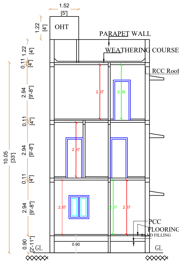
SECTION A-A
