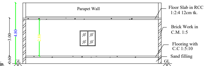
SECTION K-A
