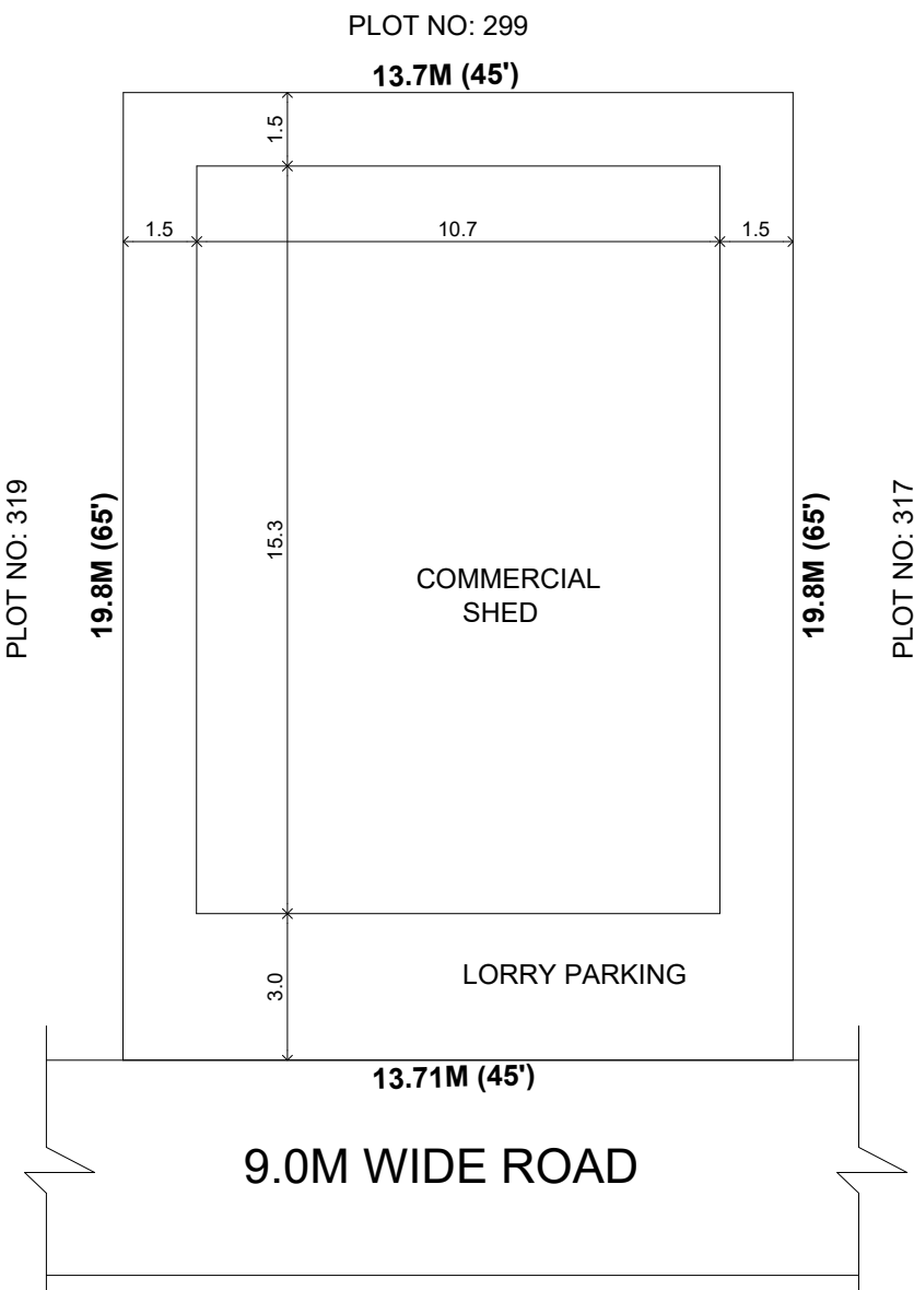
SITE PLAN 1:100
