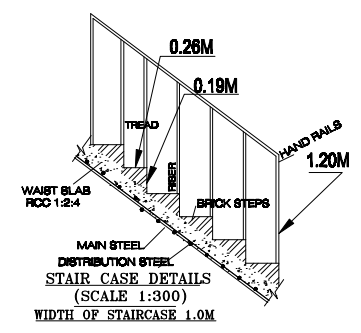
(SCALE 1:300)
