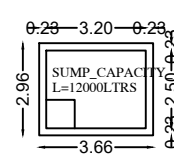
SUMP
