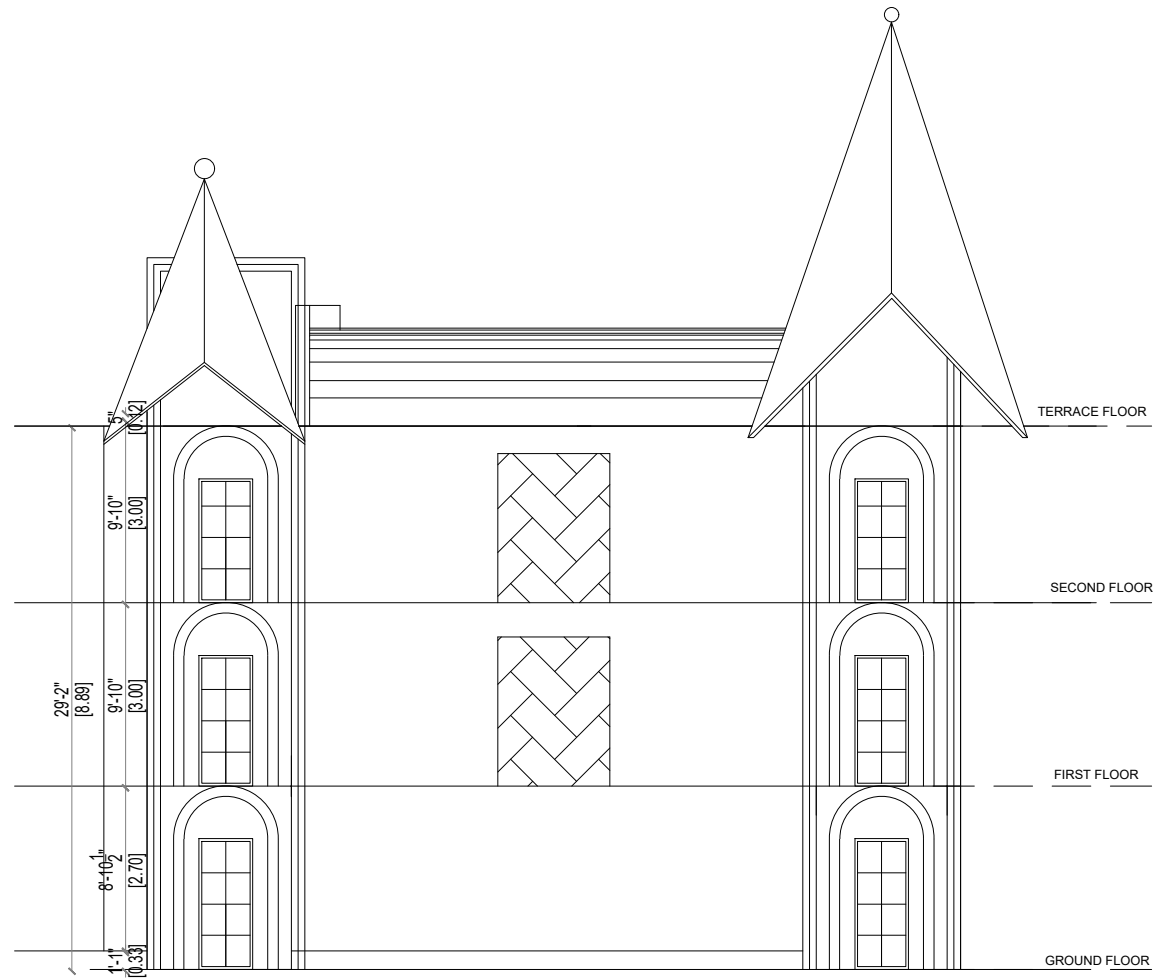
ELEVATION
