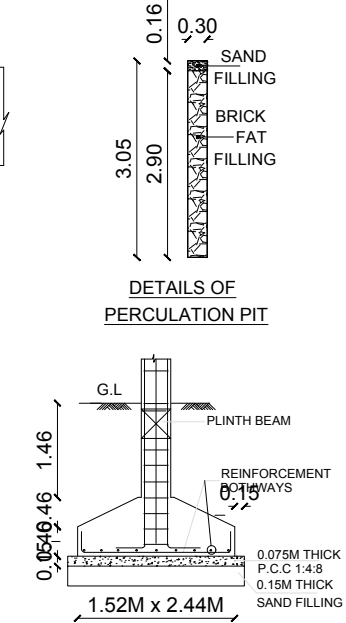
TYP. DET. COLUMN FOOTING
