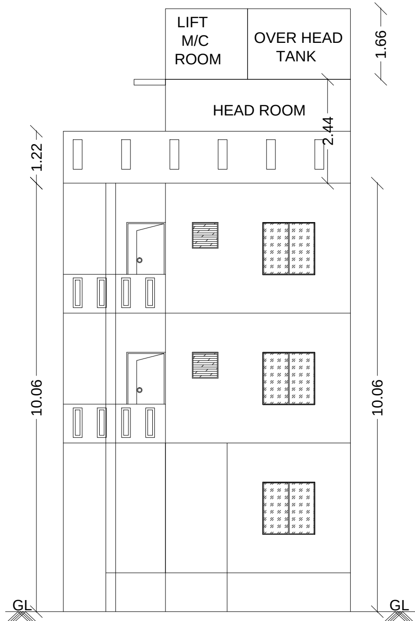
ELEVATION
