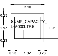
SUMP
