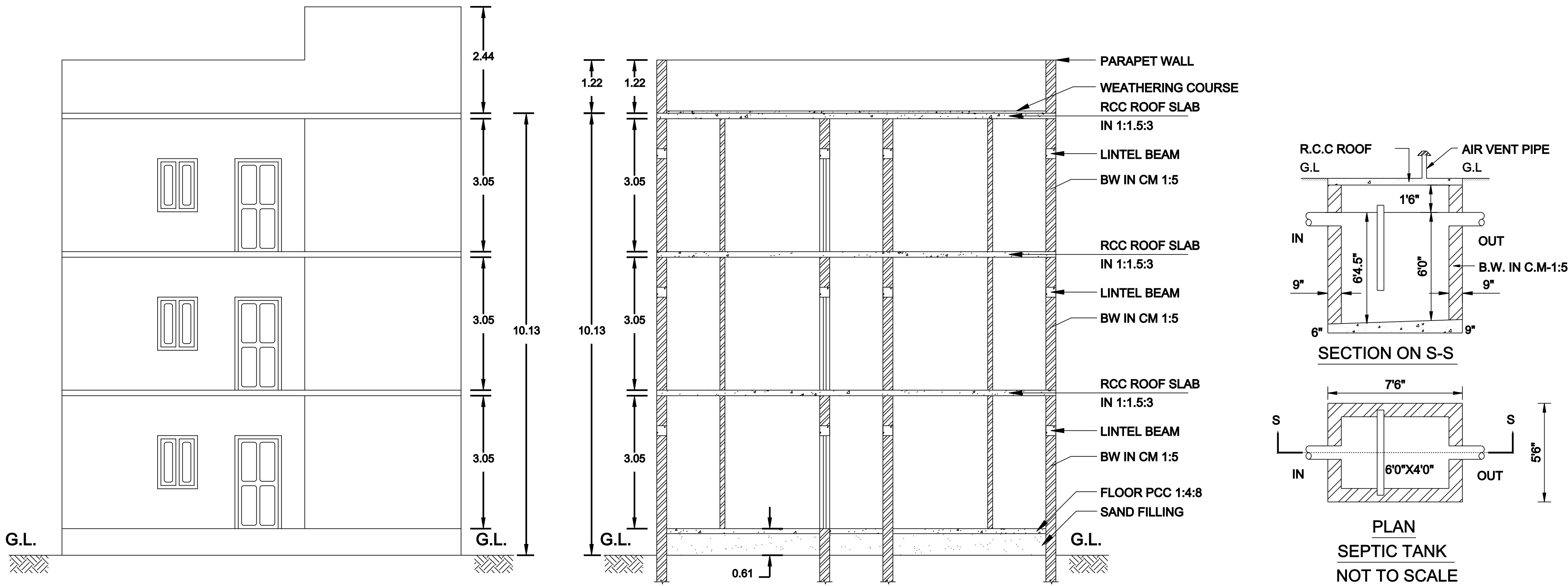
ELEVATION
