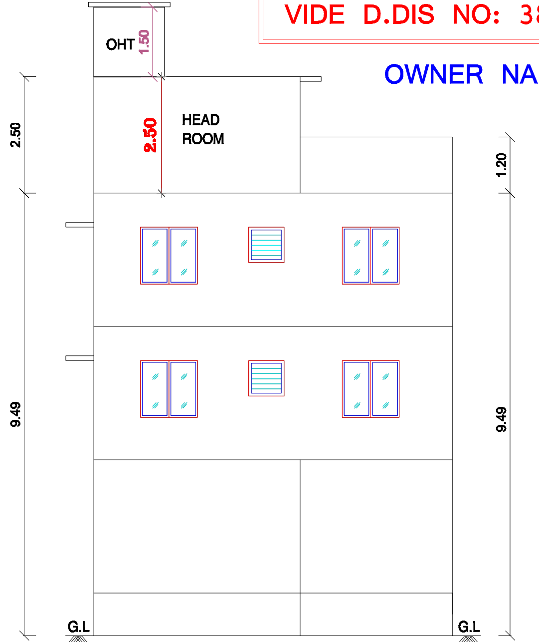
ELEVATION
