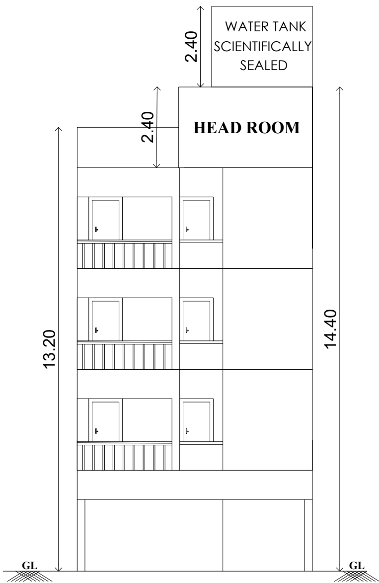
ELEVATION
