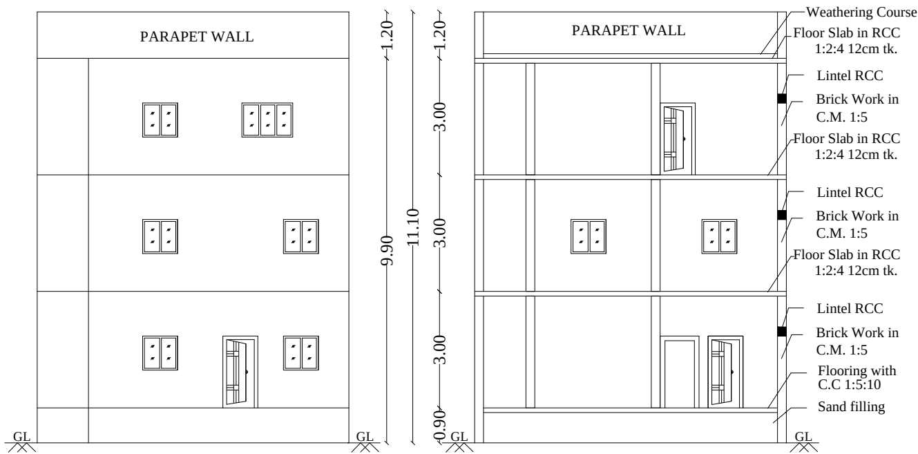
ELEVATION
